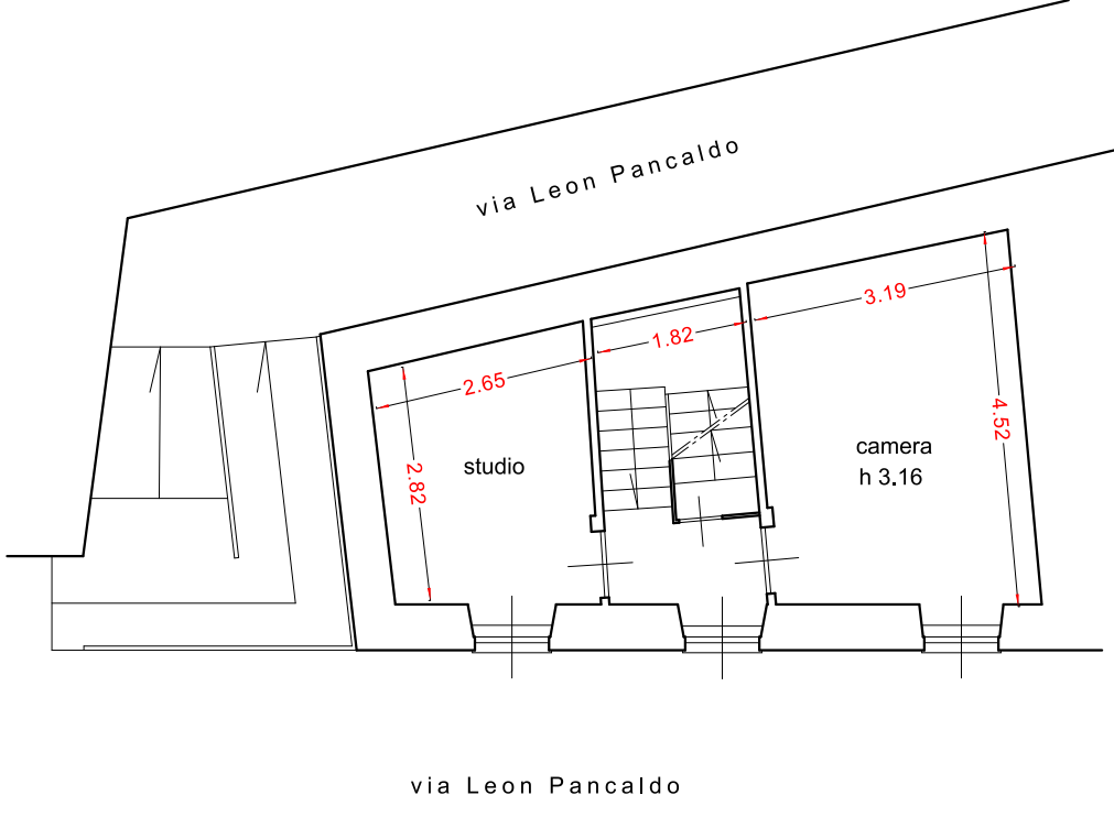
PIANO SECONDO
